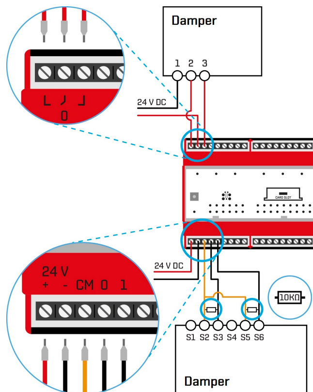
Przykład podłączenia siłownika z dwoma wyłącznikami krańcowymi
